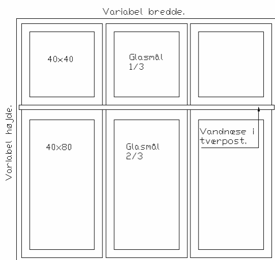
Type 5. 3-fags Dannebrogsvindue.
