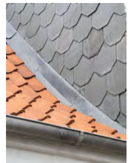
Zinkafdækning ved tag mod lodret skifervæg.
