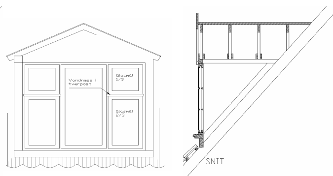
Sadelkvist set forfra og i snit.
